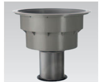
Schutz-Einlage mit integriertem Schwimmer verhindert beim Nasssaugen das Eindringen von Flüssigkeit in die Filter oder Saugmotoren
