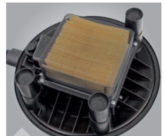
Schutz des Luftfilters vor groben Partikeln durch ein Metallgitter
